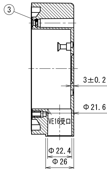
断面 A-A
